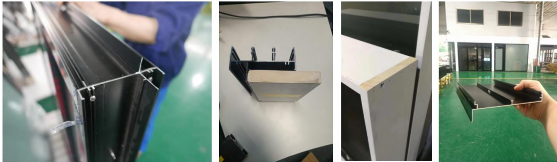
Timber reveal (Subsill+latch)
